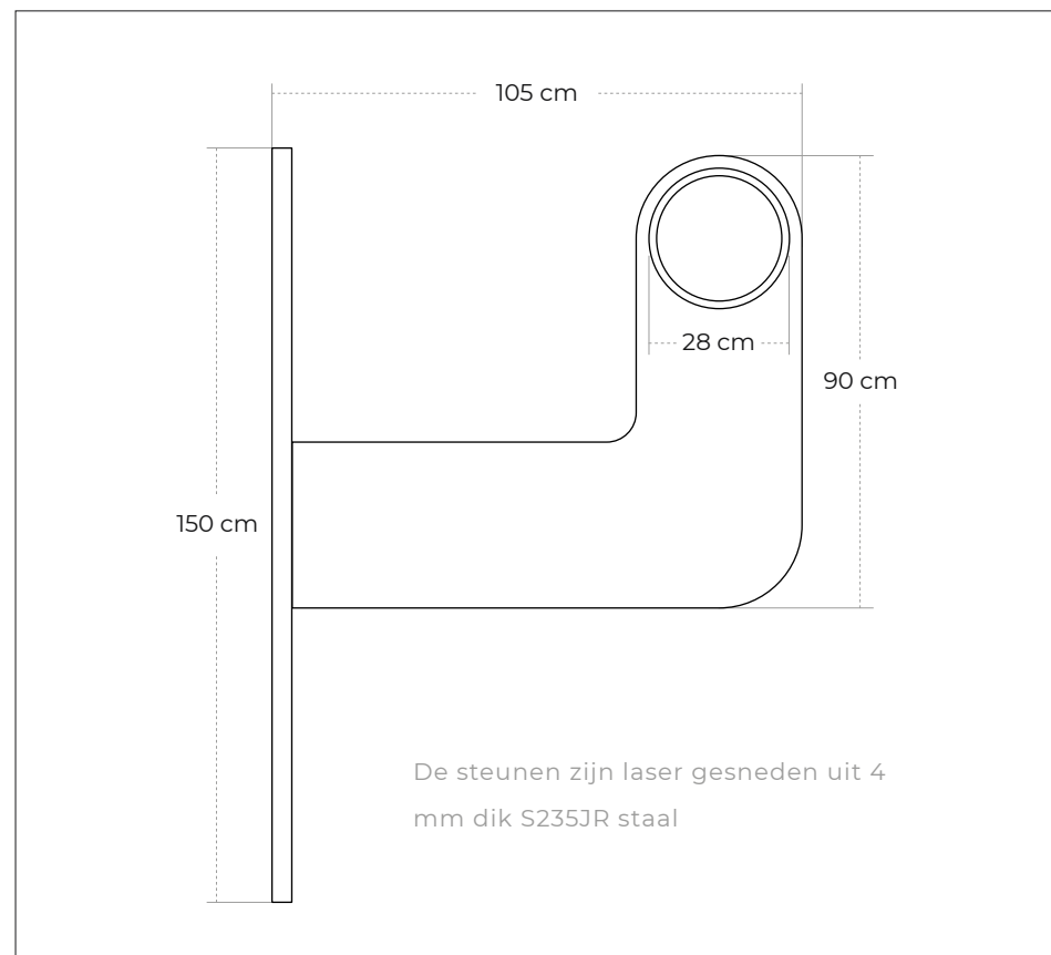
Zijaanzicht beugel
